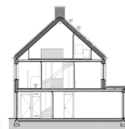
Doorsnede
