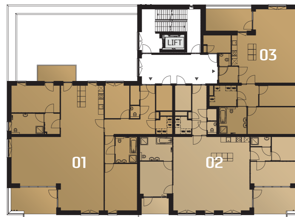
EERSTE VERDIEPING
